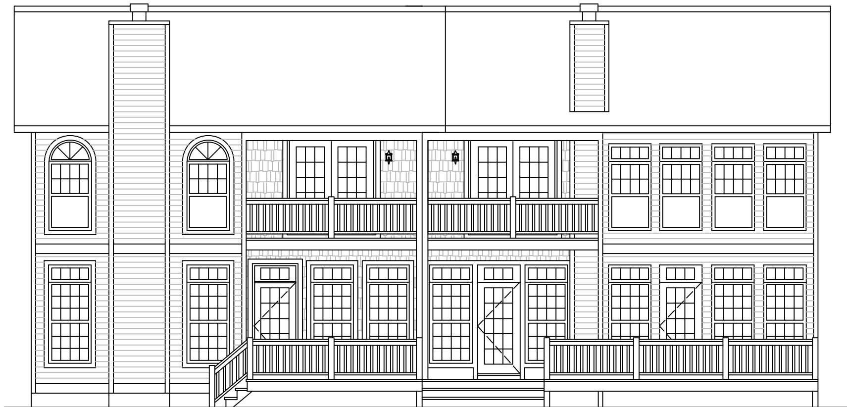
LAKE ELEVATION
